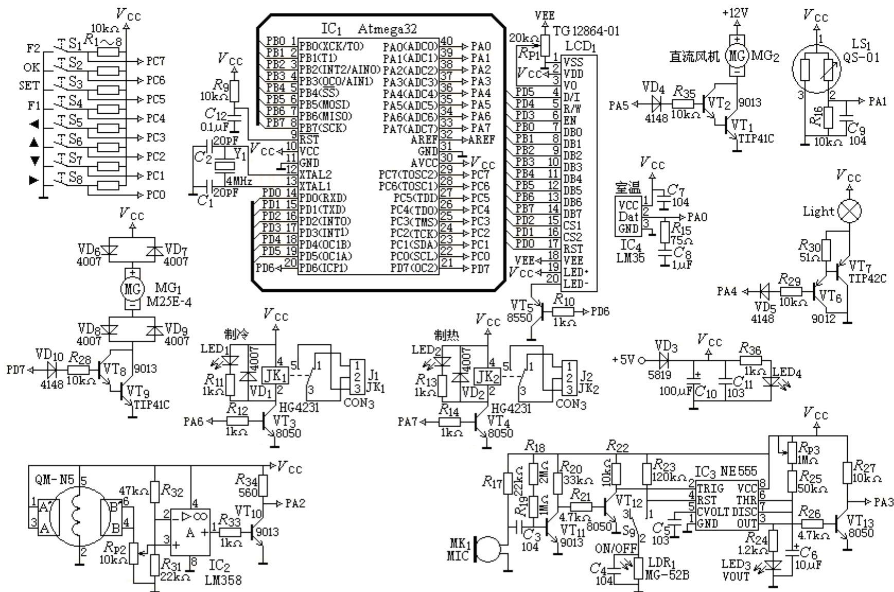
附图 1 室内家居环境控制电路图
